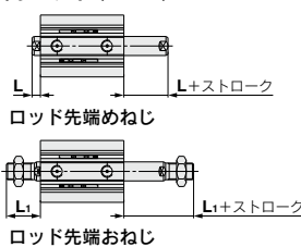
XC2A 標準形、ロッド回り止め形 (mm)
