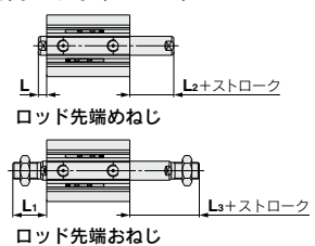
XC2A 標準形、ロッド回り止め形 (mm)
