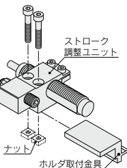
MY2H-A25L2-7-XB20 (ロングスベアサ付)
