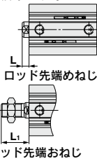
XC2 標準形、耐横荷重形、ロッド回り止め形 (mm)
