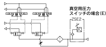
回路図
